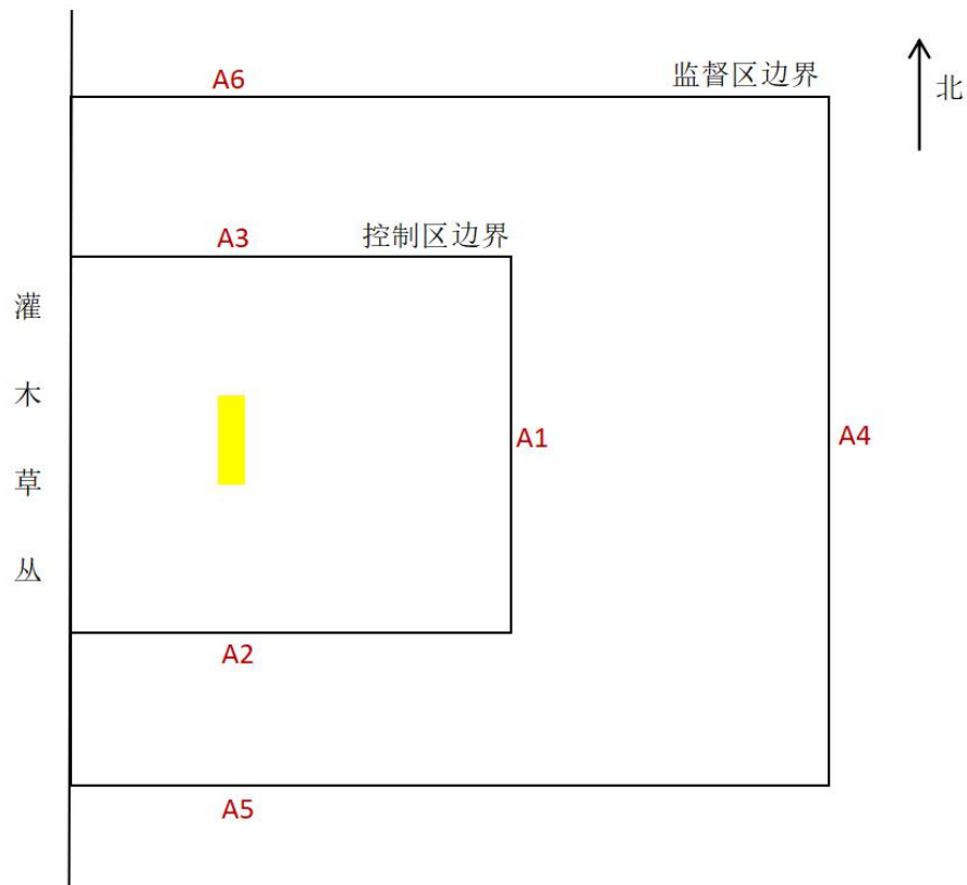
图 6-1 X 射线探伤机探伤现场检测布点示意图
