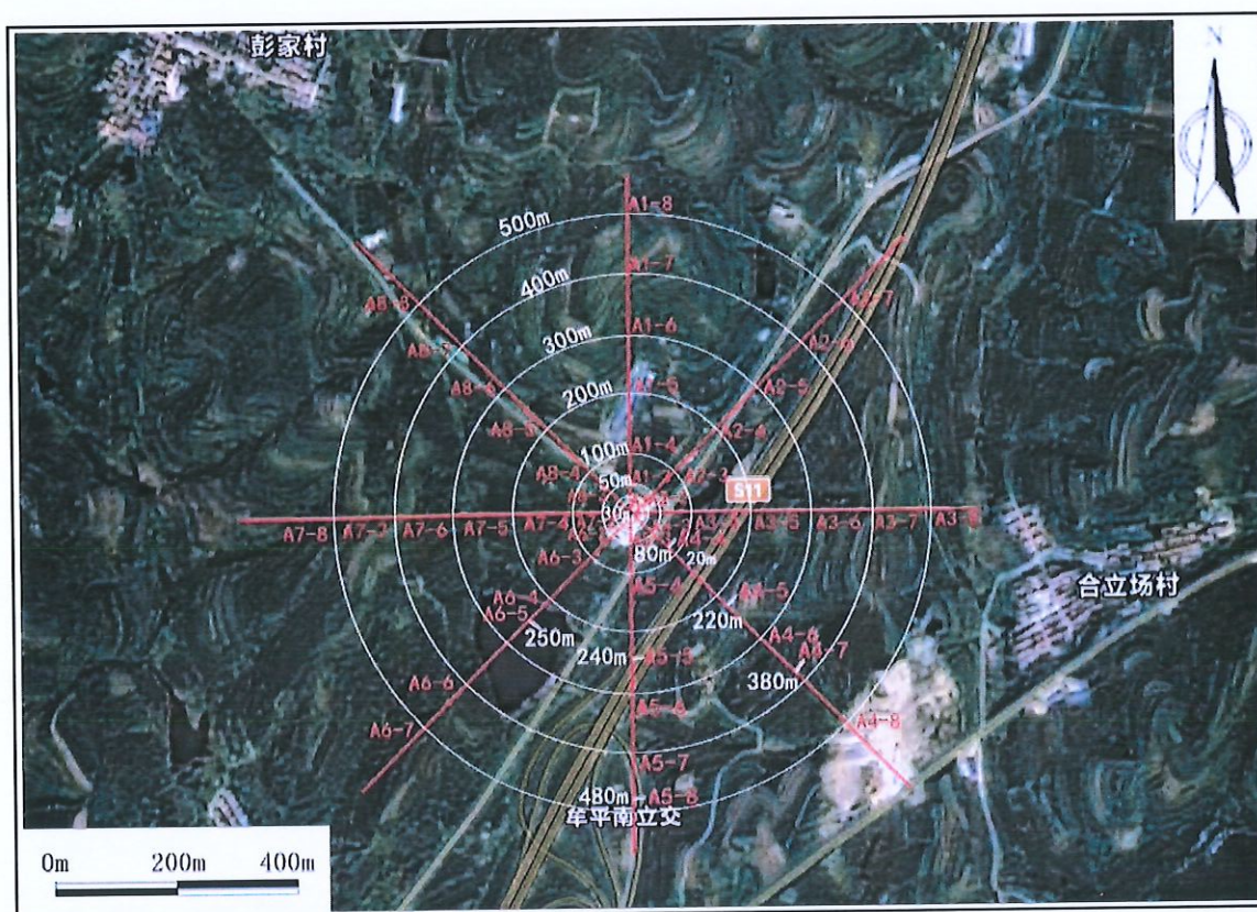
图7-1 雷达0° ~ 360° 断面监测布点示意图
