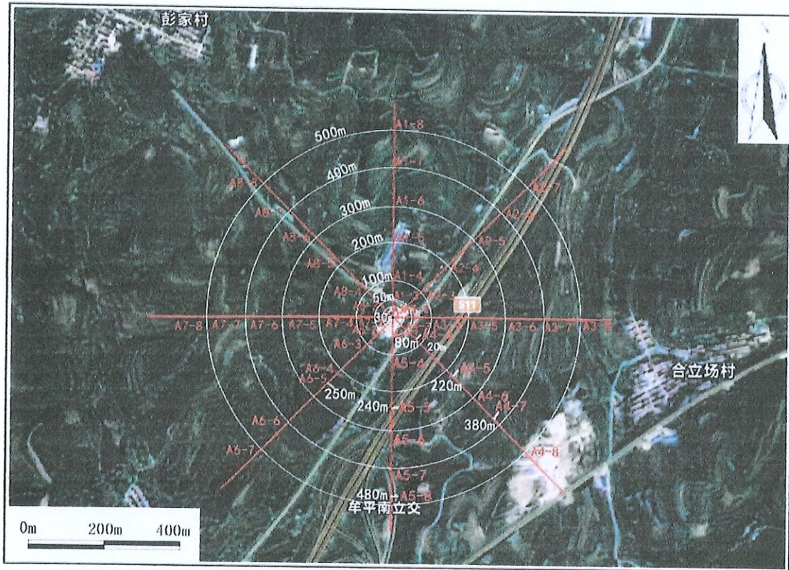
附图 2: 监测布点示意图
