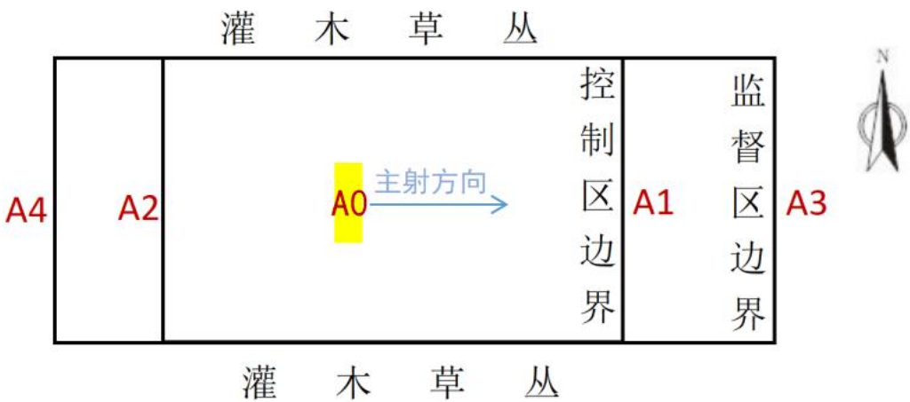
图 6-1 X 射线探伤机探伤现场检测布点示意图
