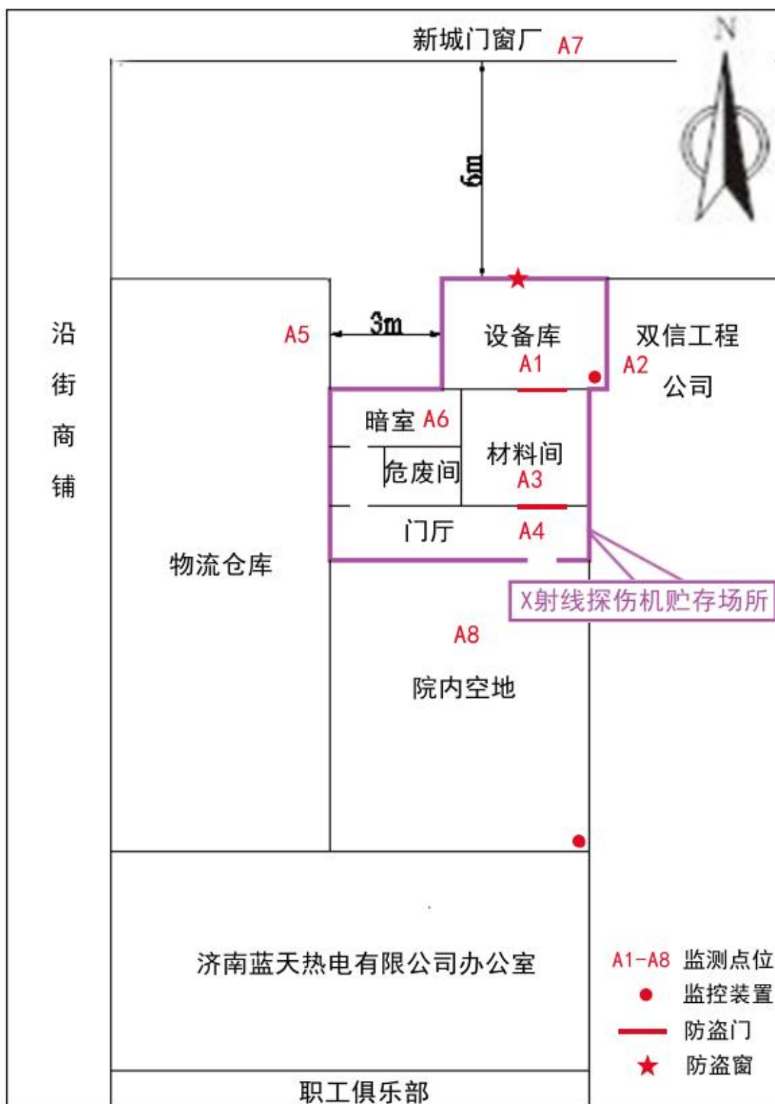
图 4-3 探伤机贮存场所平面布置示意图
