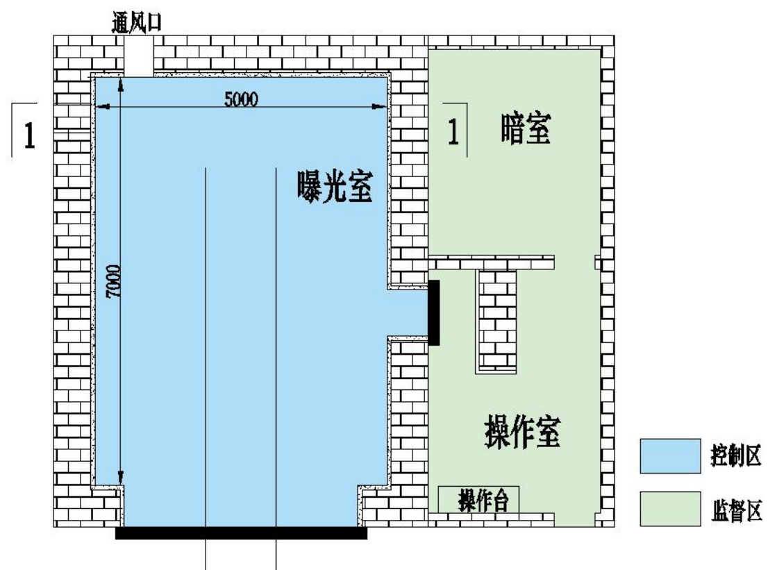
图 2-4 探伤室平面布置示意图
