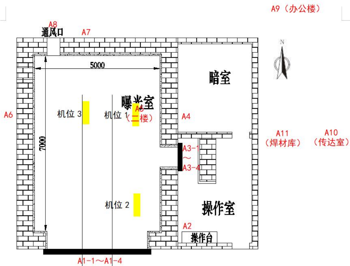
图 5-1 探伤室监测点位示意图
