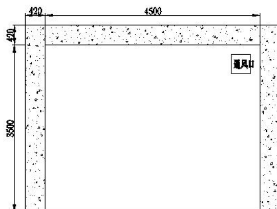
图2-4 (b) 探伤室1-1剖面示意图
