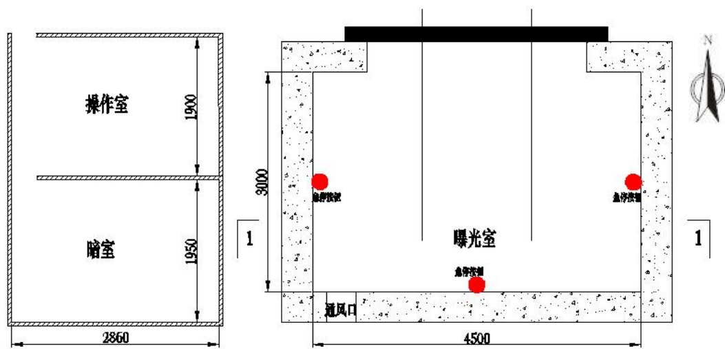
图 2-4 (a) 探伤室平面布置示意图
