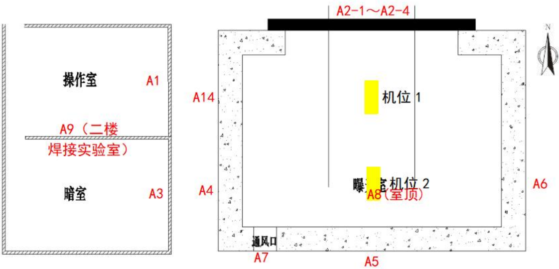
图 5-1 探伤室监测点位示意图
