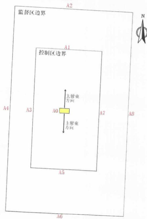
附图 1: 模拟探伤现场检测点位示意图
