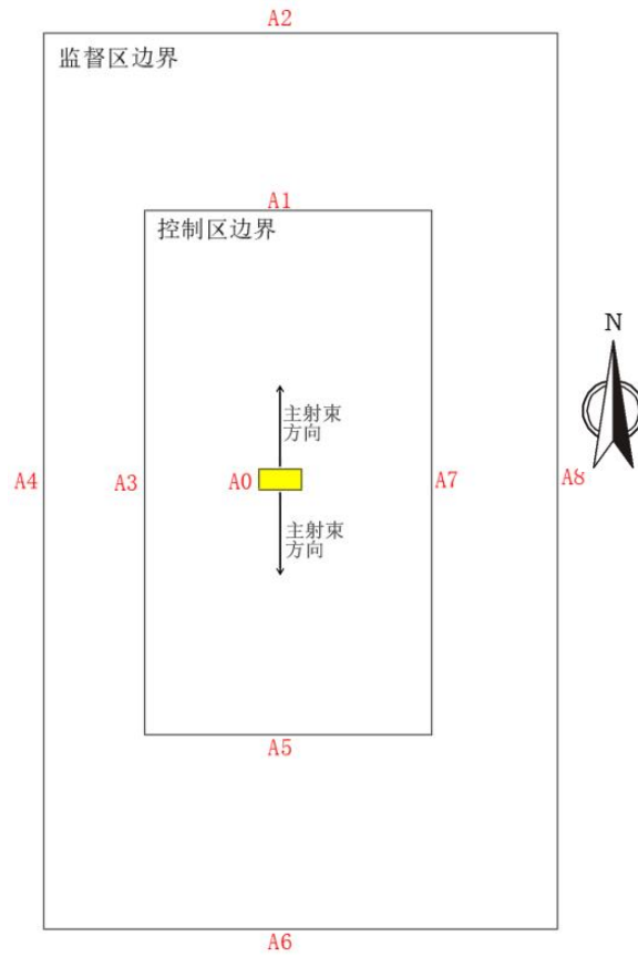
图 6-1 监测布点图
