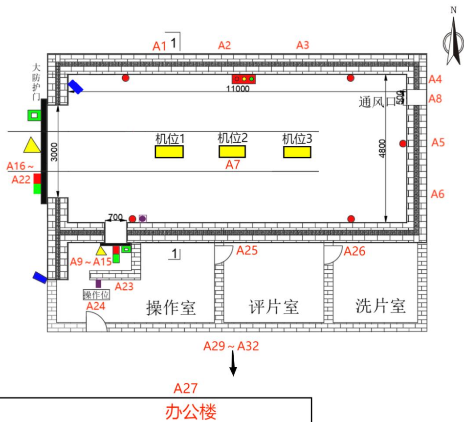
图 6-1 监测布点图
