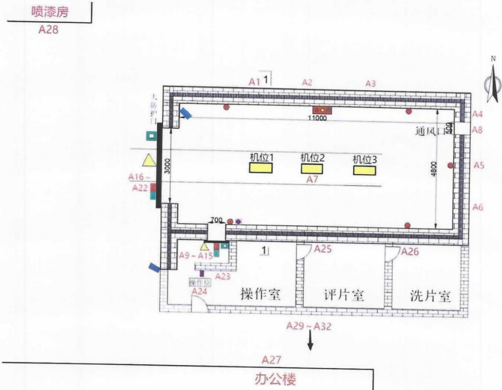
附图 1: 检测布点示意图
