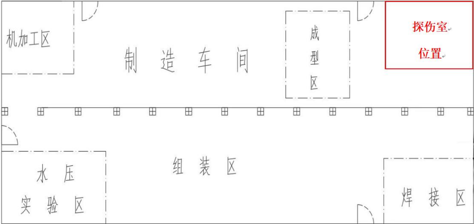
附图四：山东宏达科技集团有限公司五峰厂区制造车间平面布置示意图
