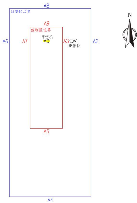
图 6-1 XXG-1605 型探伤机检测布点示意图
