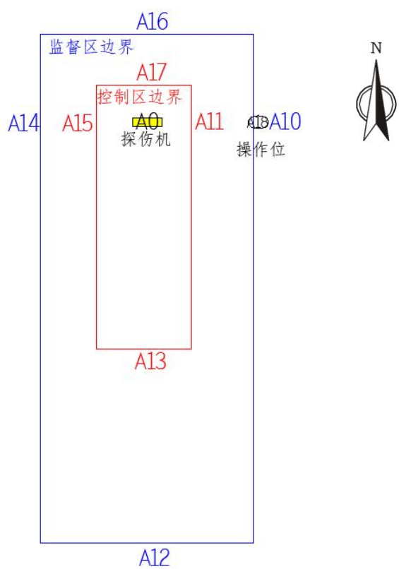
图 6-2 XXG-2505 型探伤机检测布点示意图
