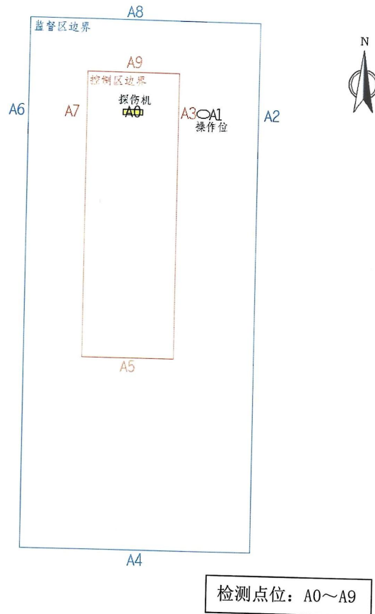
附图 1：XXG-1605 型 X 射线探伤机检测布点示意图
