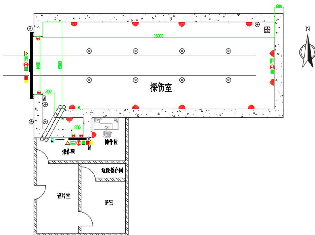
图 3-2 验收探伤场所布局图 (mm)
