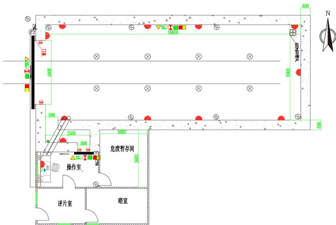
图 3-1 环评探伤场所布局图 (mm)
