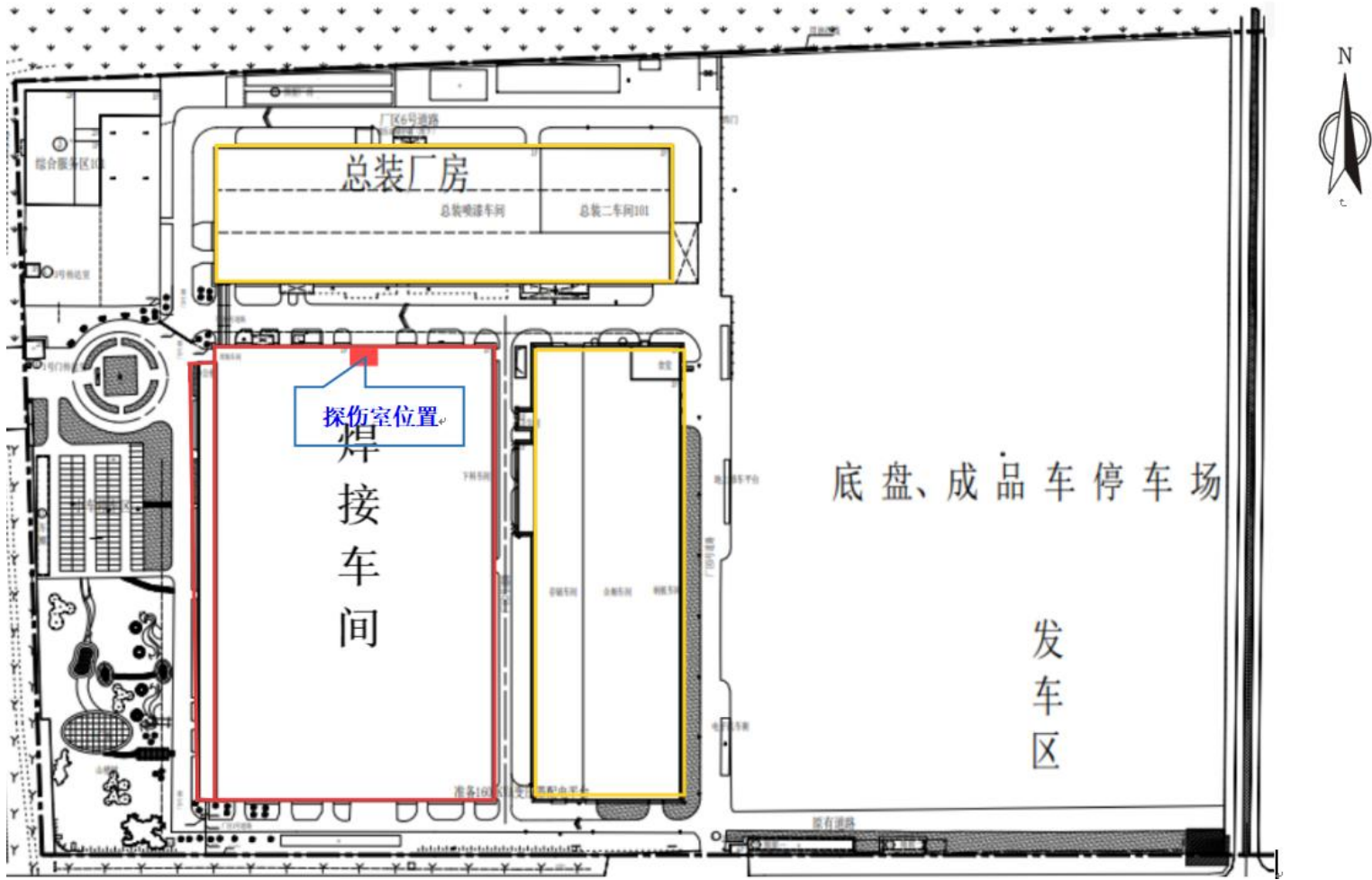
附图三 中国重汽集团济南专用车有限公司总平面图
