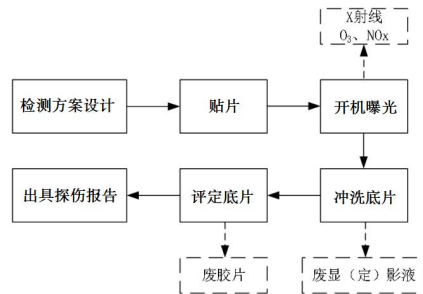
图 2-4 X 射线探伤机工作流程示意图
