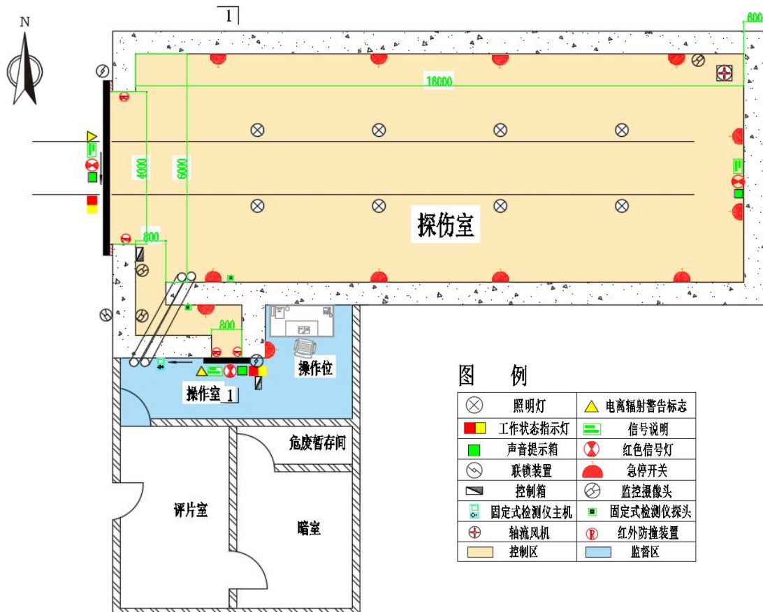
图 2-1 (a) 本项目探伤室平面布置图 (单位: mm)
