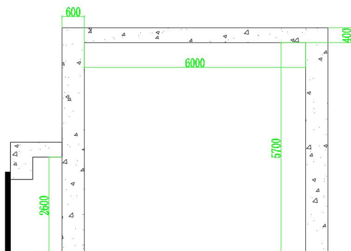
图 2-1 (b) 1-1 剖面布置图 (单位: mm)
