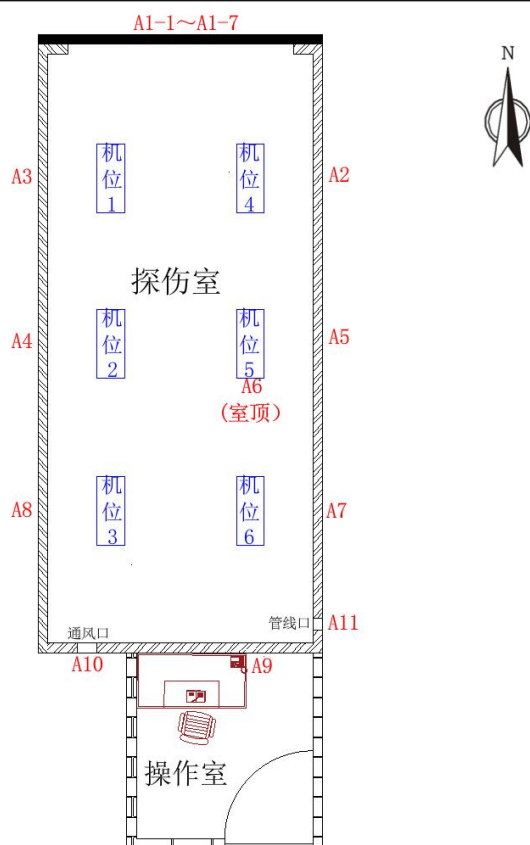
图 6-2 (a) 工作状态监测布点图
