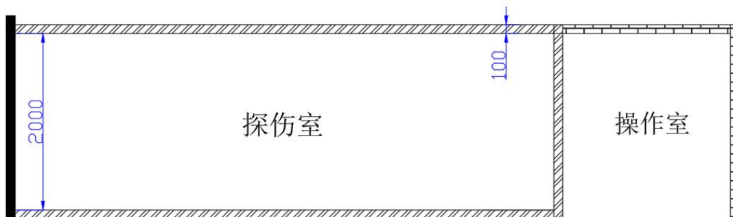
图 2-1 (b) 本项目探伤室 1-1 剖面布置图 (mm)
