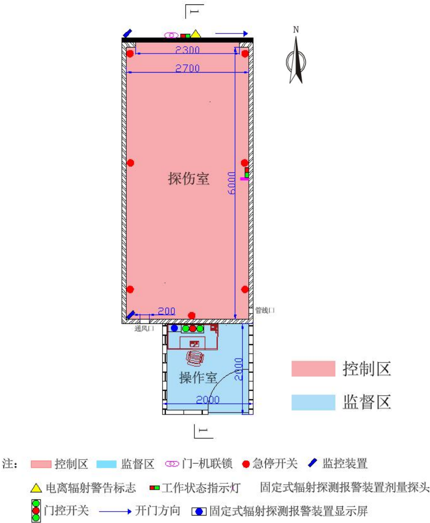
图 2-1（a） 本项目探伤室平面布置图（mm）
