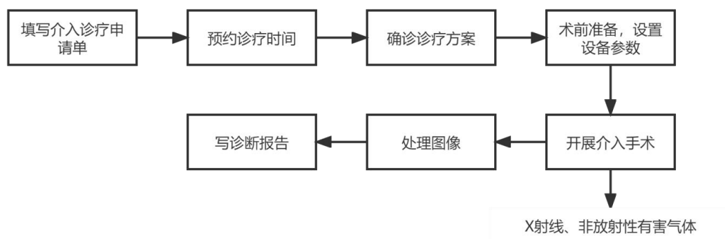
图 2-3 介入诊断工艺流程及产污环节图
