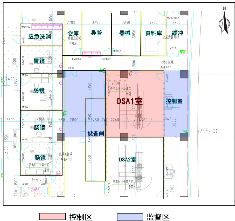
图 2-2 DSA 工作场所平面布置图
