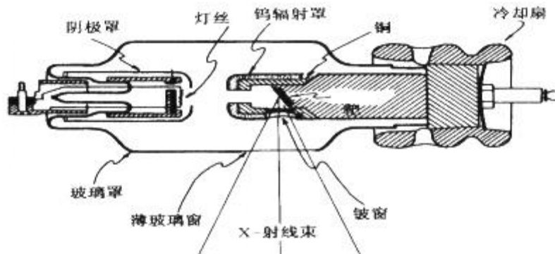
图 2-3 典型 X 射线管结构图
